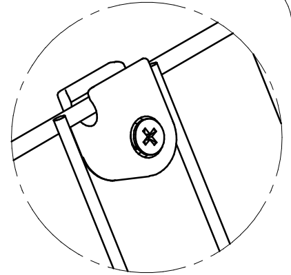
DETT. B
